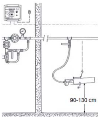
Fig 1: Central control brooding system can be applied using conventional propane gas cylinder. 图1: 中央控制育雏系统，可以采用传统的丙烷气瓶。
